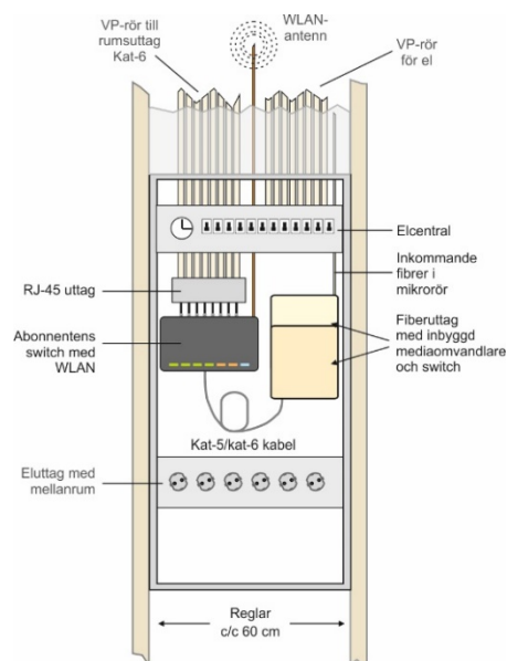
Exempel på bredbandsutrymme kombinerat med elcentral i bostad
