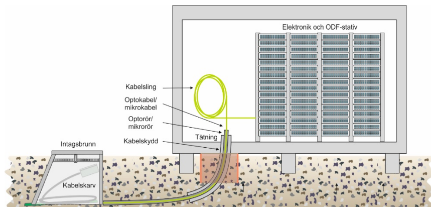
Exempel på intagsbrunn
