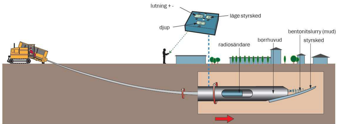
Exempel styrd borrar
