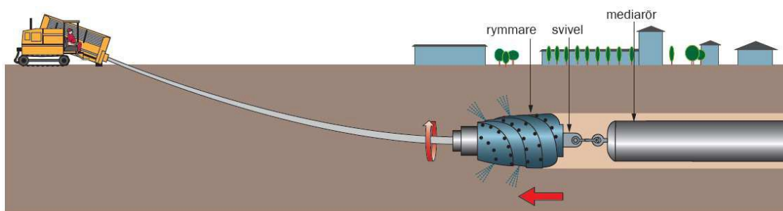
Exempel styrd borrarling när mediaröret (kanalisationsrör) dras tillbaka med rymmare.
