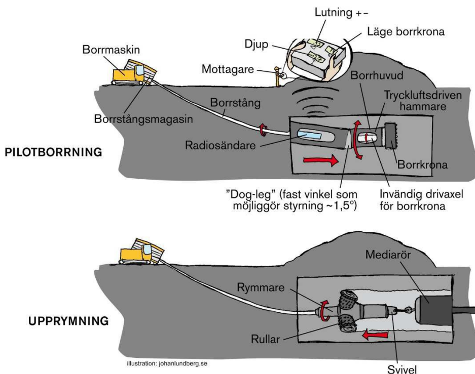
Illustration som visar AT- borrning
