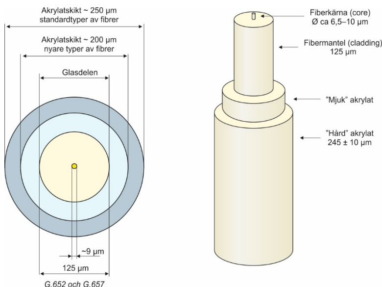
Bild uppbyggnad av optokabel .652 och .657.
