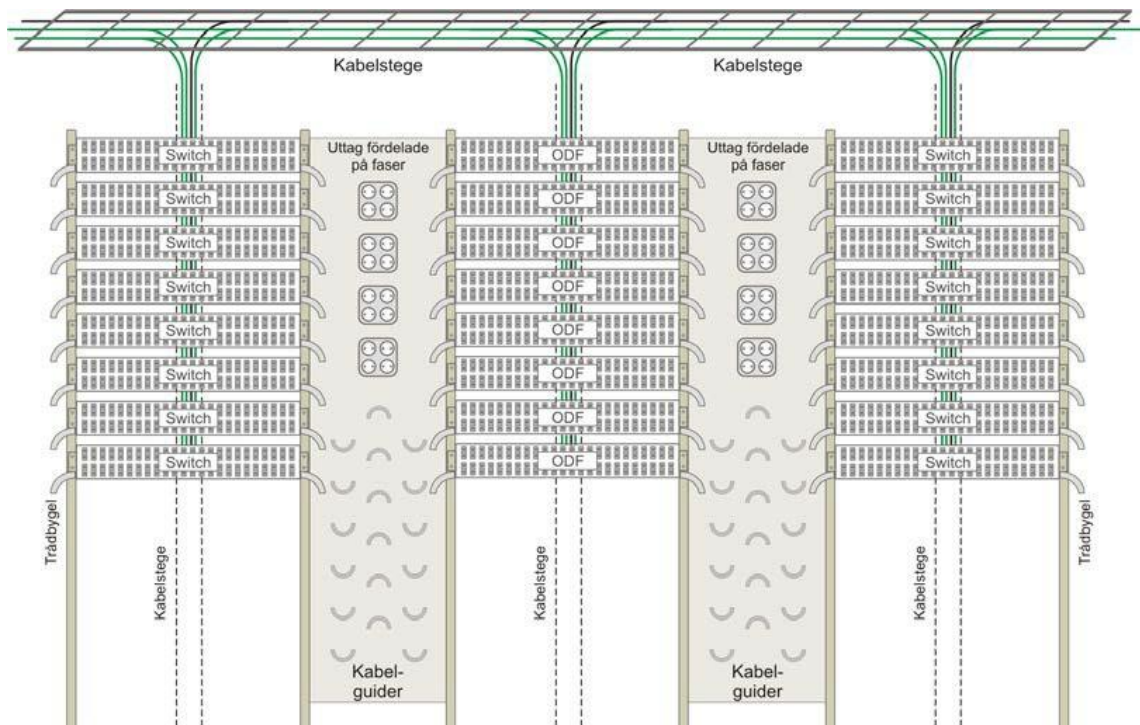
Exempel på stativplacering
