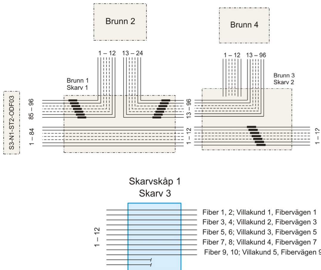
Exempel skarvplan
