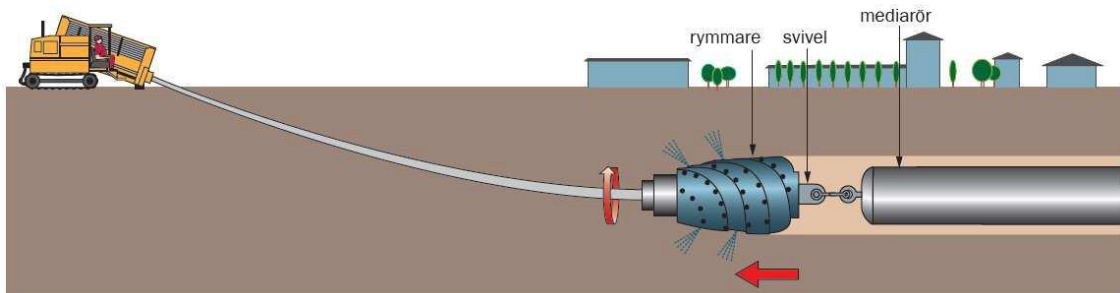
Exempel styrd borrarbete när mediaröret (kanalisationsrör) dras tillbaka med rymmaren.
