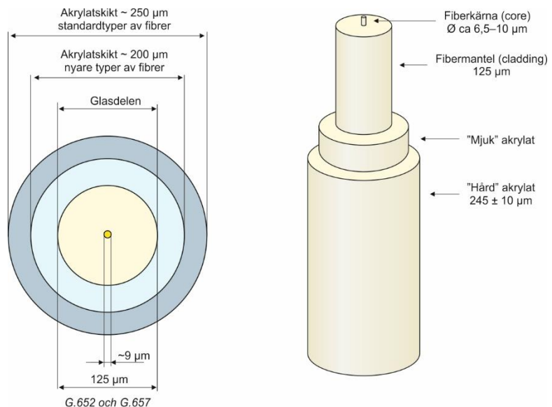
Bild uppbyggd av fiber i optokabel G.652 och G.657.
