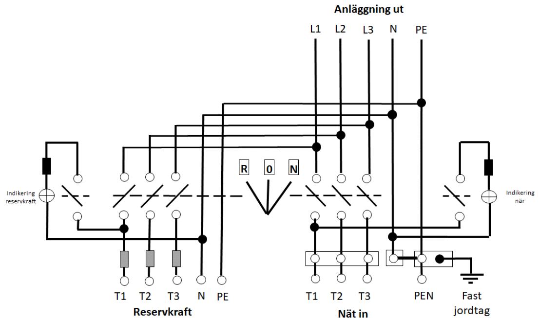
Bild. Kopplingsschema för anslutning av reservverk site
