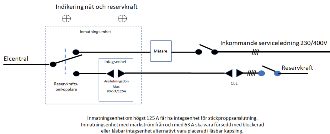
Bild. Princip för anslutning av reservkraft i site
