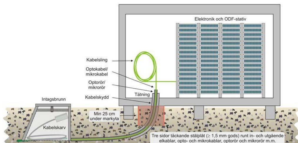
Exempel kabelintag
