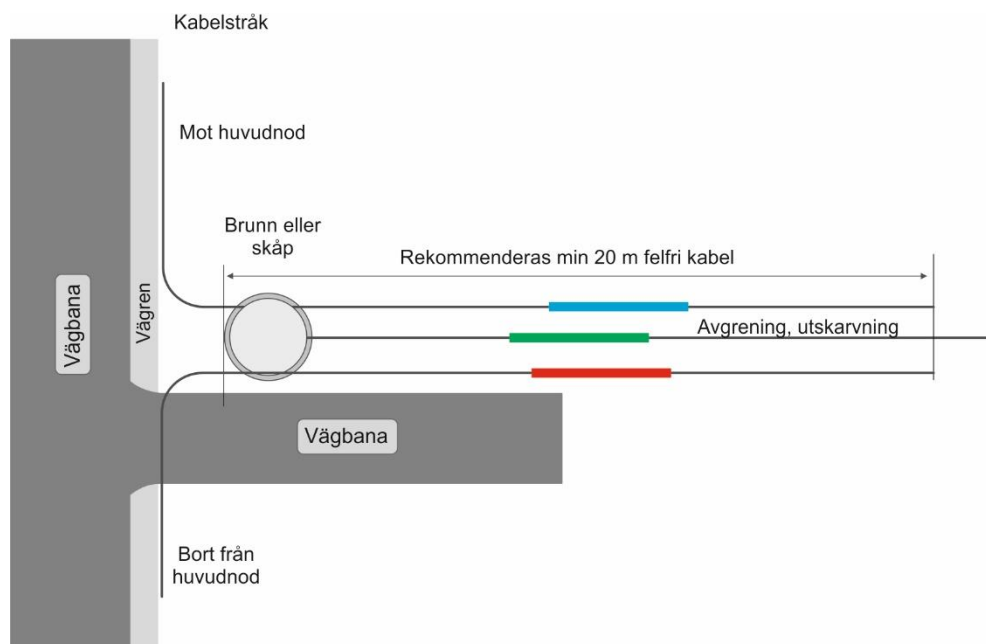
Exempel på märkning av kablar i brunnar och skåp
