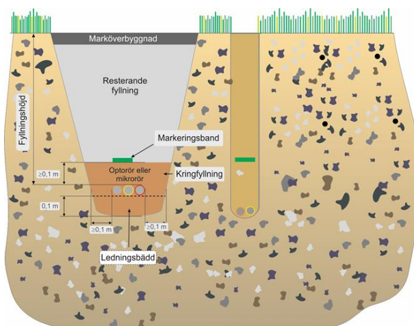
Exempel på ledningsbädd och kringfyllning
