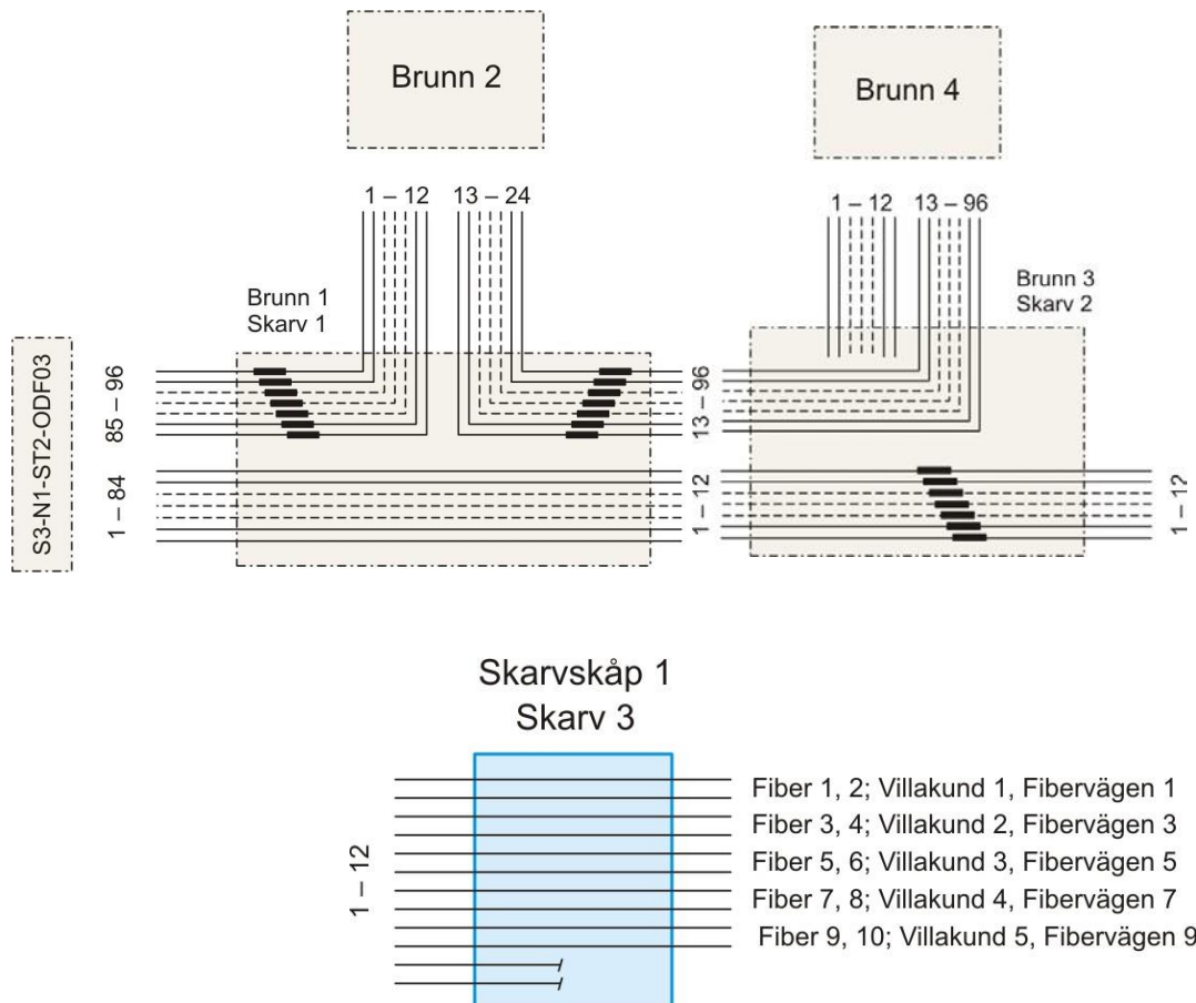
Exempel skarvplan
