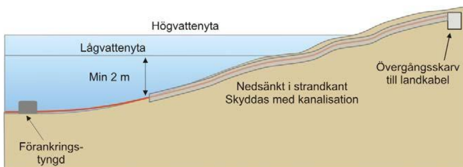
Exempel visar förläggning av kanalisering 2 m under lågvattenyta
