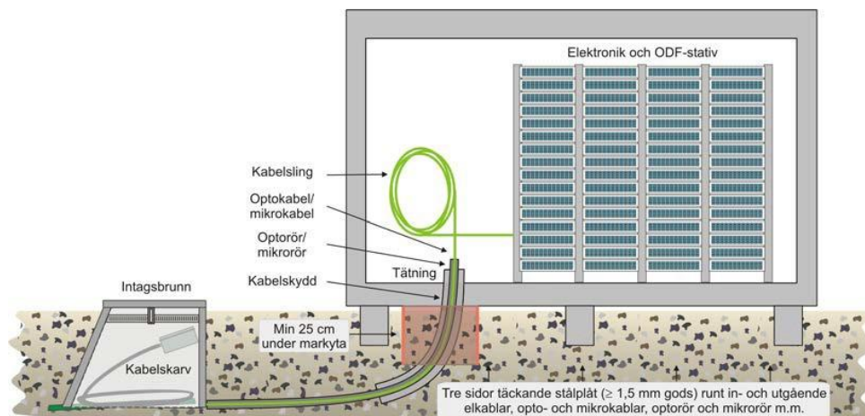
Exempel kabelintag
