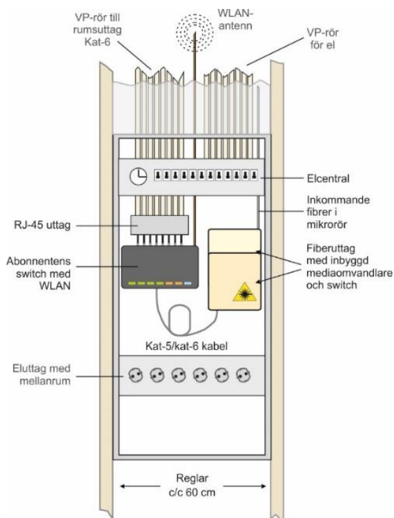
Exempel på broadbandutrymme kombinerat med elcentral i bostad.
