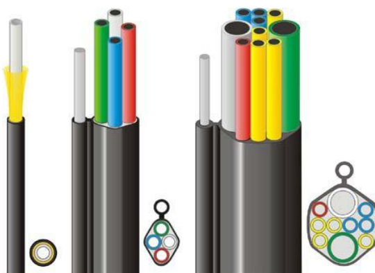
Mikrorör för luftförläggning.
